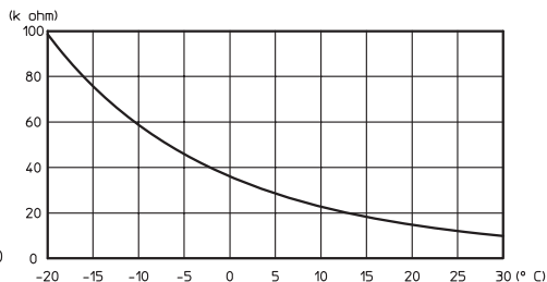
2. ábra: az érzékelő karakterisztikája 3.015266, 35 kW feletti kazánok
