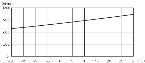
1. ábra: az érzékelő karakterisztikája 3.014083, 35 kW alatti kazánok
