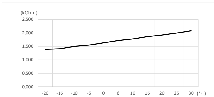
3. ábra: az érzékelő karakterisztikája 3.024511, kaszkádszabályzóhoz
