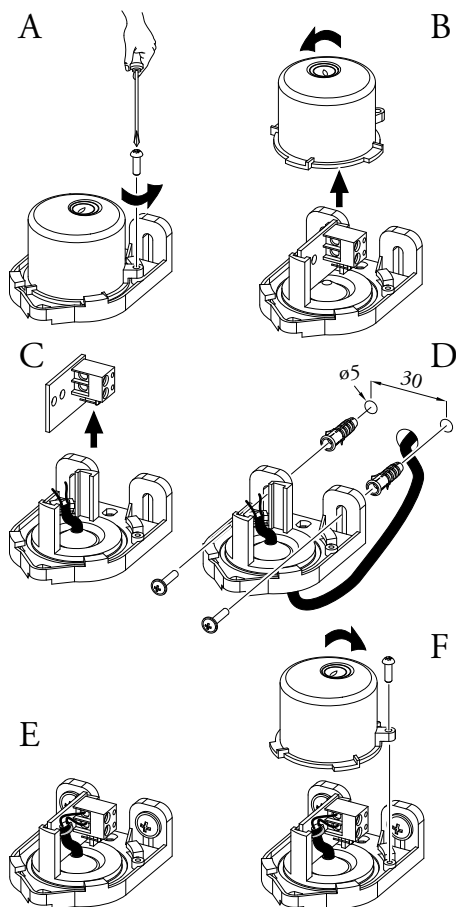
4. ábra: vízszintes elhelyezés
